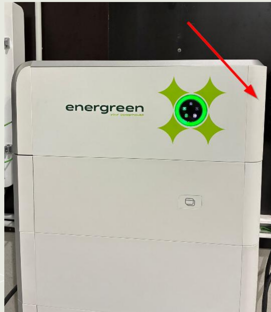
STAP 2: Vervolgens dient u de rechterkap te demonteren. Dit kan u doen door de kap naar boven te schuiven.
